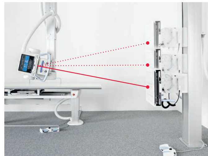
Das Stitching (Wand oder Tisch) ist komplett in die Bedienoberfläche integriert und automatisiert. Das Röntgensystem unterstützt dabei das Einrichten graphisch, berechnet die benötigte Anzahl Bilder selbstständig und verfährt die gesamte Aufnahme automatisch.
